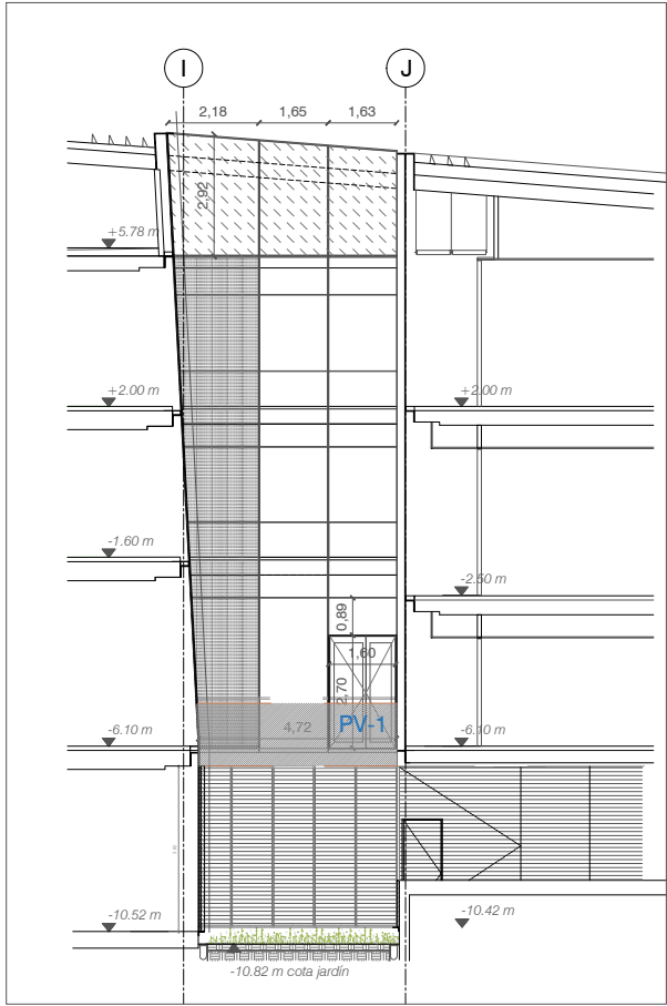
SECCIÓN C-C MC-1
