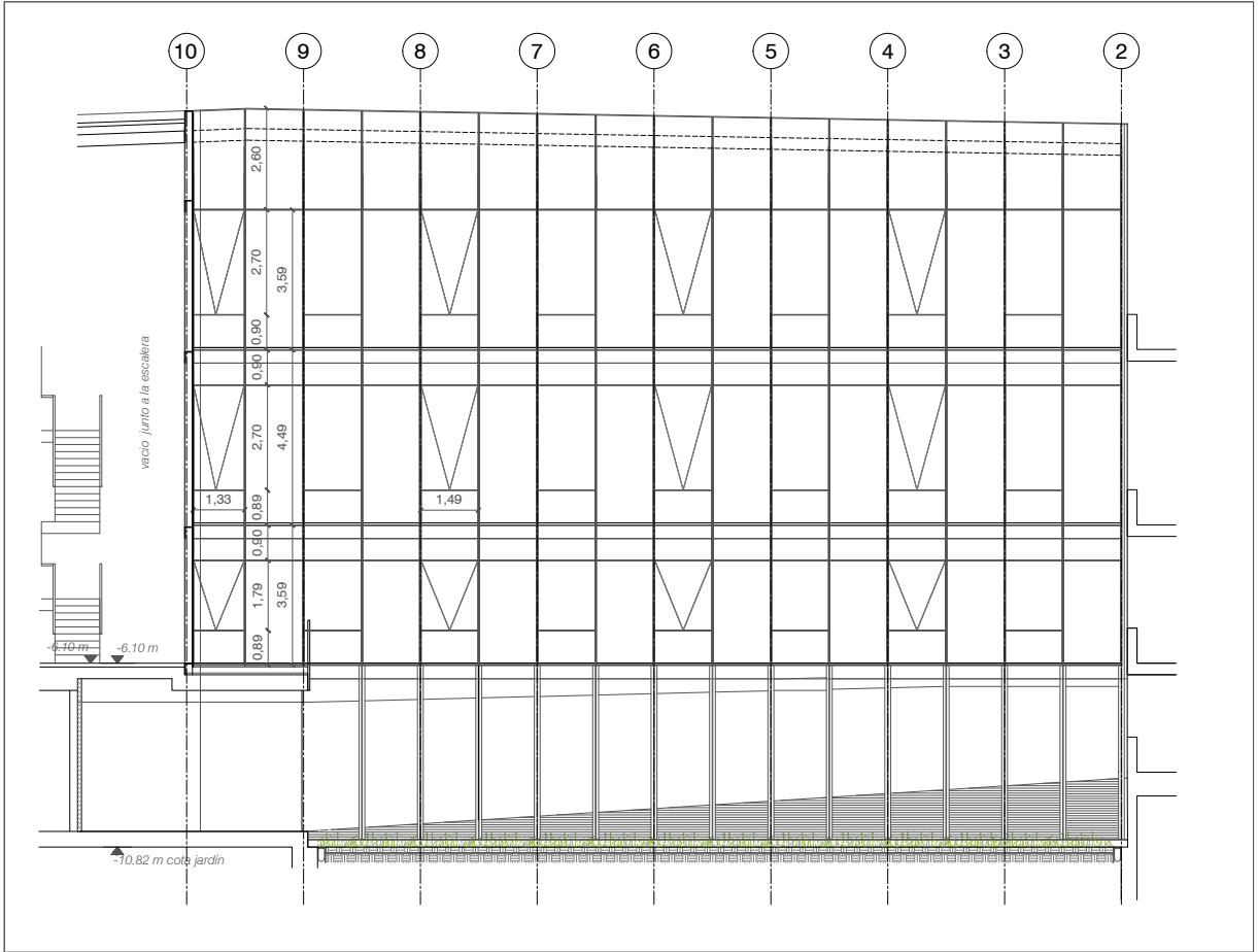
SECCIÓN B-B MC-1
