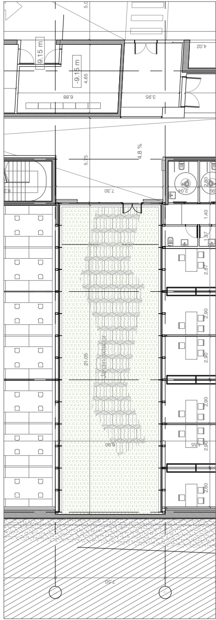
PLANTA SEMISÓTANO
