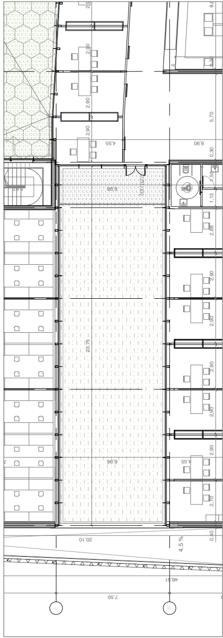
PLANTA BAJA
