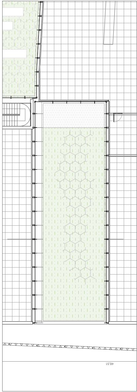
PLANTA INSTALACIONES
