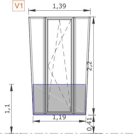
tipo: V1 60 unidades apertura: 1 hoja oscilobatiente, 2 fijos laterales medidas: 1,19 x 2,20m material: aluminio anodizado plata vidrio bajo emisivo laminar 4/18/4.4 al interior * ubicación: fachada sur plantas 1ª a 6ª barandilla al exterior de vidrio laminar
