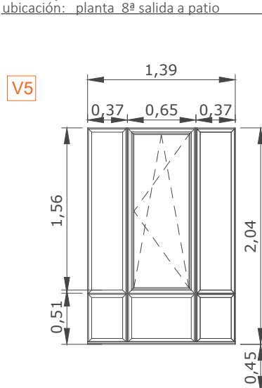
tipo: V5 77 unidades apertura: 1 hoja oscilobatiente, fijo lateral e inferior medidas: 1,39 x 2,04m material: aluminio anodizado plata vidrio bajo emisivo laminar 4/18/4.4 al interior * ubicación: en fachada norte de planta 1ª a 7ª, en fachada sur planta 7ª
