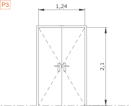
tipo: P3 1 unidad apertura: 2 hojas abatibles medidas: 0,62 x 2,10m material: tablero MDF ubicación: planta tercera entrada a puestos de trabajo
