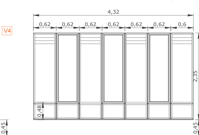
tipo: V4 8 unidades apertura: 3 hojas oscilobatientes, fijo inferior y lateral medidas: 4,32 x 2,35m material: aluminio anodizado plata, cristal al ácido vidrio bajo emisivo laminar 4/18/4.4 al interior ubicación: en fachada medianera de planta 1ª a 8ª
