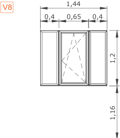
tipo: V8 10 unidades apertura: 1 hoja oscilobatiente, fijos laterales medidas: 1,44 x 1,20m material: aluminio anodizado plata vidrio bajo emisivo: 6+18+6 ubicación: planta 8ª fachada norte
