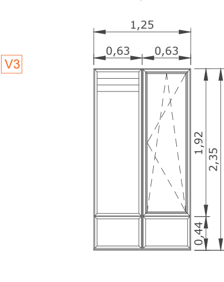
tipo: V3 8 unidades apertura: 1 hoja oscilobatiente, fijo inferior y lateral medidas: 1,25 x 2,35m material: aluminio anodizado plata, cristal al ácido vidrio bajo emisivo laminar 4/18/4.4 al interior ubicación: en fachada medianera de planta 1ª a 8ª
