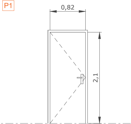
tipo: P1 133 unidades apertura: 1 hoja abatible medidas: 0,82 x 2,10m material: tablero MDF lacado en blanco ubicación: despachos, baños, almacenes, pasillos....
