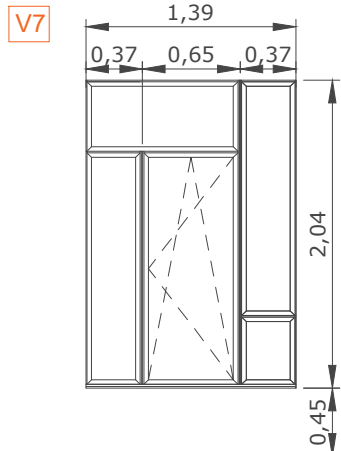
tipo: V7 3 unidades apertura: 1 hoja oscilobatiente, fijo lateral e inferior y superior medidas: 1,39 x 2,04m material: aluminio anodizado plata vidrio bajo emisivo: 4.4+18+4.4 6+18+6 en fijo superior ubicación: en fachada sur de planta 7ª
