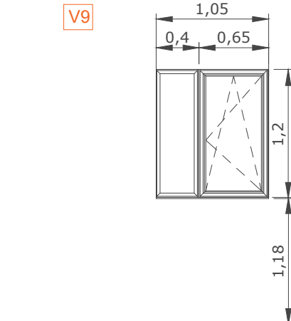
tipo: V9 2 unidades apertura: 1 hoja oscilobatiente, fijo lateral medidas: 1,05 x 1,20m material: aluminio anodizado plata vidrio bajo emisivo: 6+18+6 ubicación: planta 8ª fachada norte
