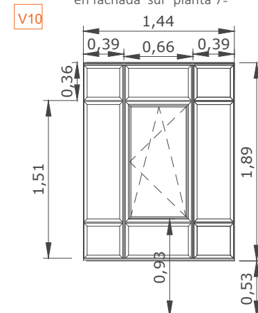
tipo: V10 14 unidades apertura: 1 hoja oscilobatiente, fijos laterales superiores e inferiores medidas: 1,44 x 1,89m material: aluminio anodizado plata vidrio bajo emisivo: 4.4+18+4.4 ** ubicación: planta 8ª fachada a patio
