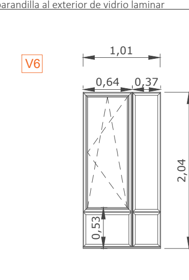
tipo: V6 16 unidades apertura: 1 hoja oscilobatiente, fijo lateral e inferior medidas: 1,01 x 2,04m material: aluminio anodizado plata vidrio bajo emisivo laminar 4/18/4.4 al interior * ubicación: en fachada norte de planta 1ª a 7ª, en fachada sur planta 7ª
