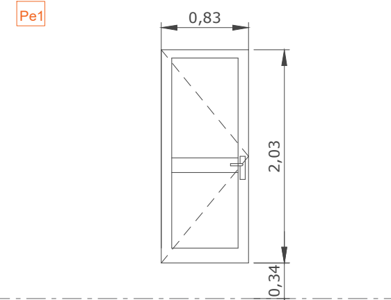
tipo: Pe1 1 unidad apertura: puerta balconera abatible medidas: 0,83 x 2,03m material: aluminio anodizado plata vidrio bajo emisivo laminar 4.4/18/4.4 ubicación: planta 8ª salida a patio
