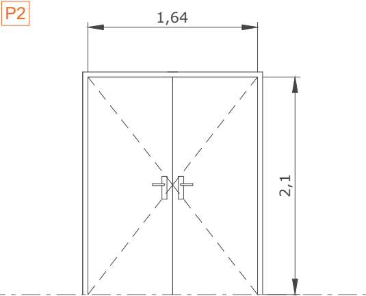
tipo: P2 15 unidades apertura: 2 hojas abatibles medidas: 0,82 x 2,10m material: tablero MDF ubicación: vestíbulos y salas de reunión
