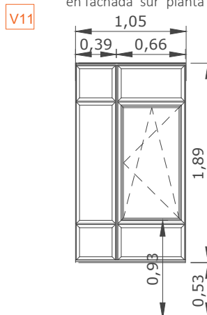
tipo: V11 2 unidades apertura: 1 hoja oscilobatiente, fijos laterales superiores e inferiores medidas: 1,05 x 1,89m material: aluminio anodizado plata vidrio bajo emisivo: 4.4+18+4.4 ** ubicación: planta 8ª fachada a patio
