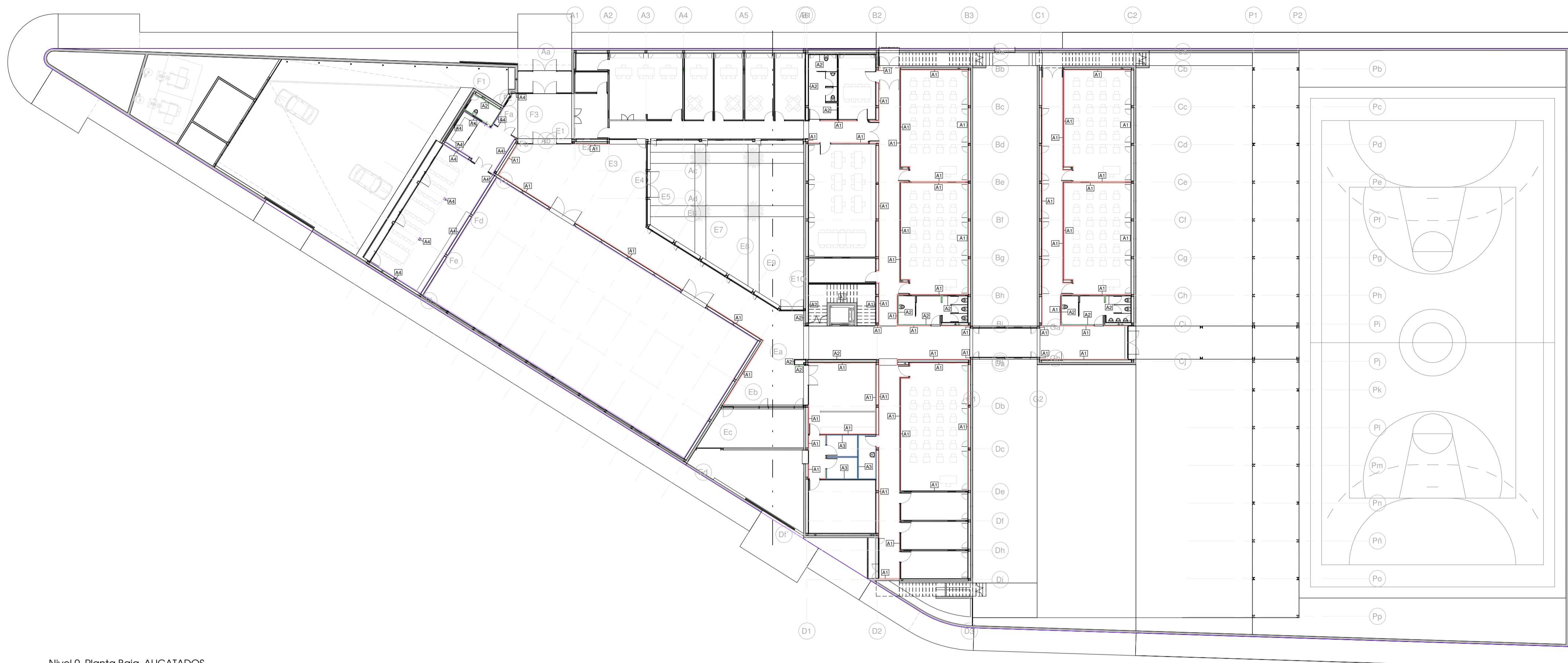
Nivel 0_Planta Baja_ALICATADOS 1 : 250
