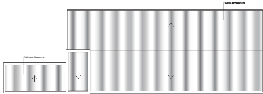
PLANTA de CUBIERTAS E:1/100
