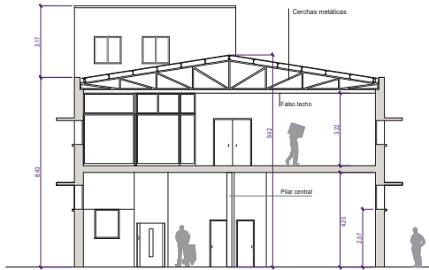
SECCIÓN S1 E:1/100
