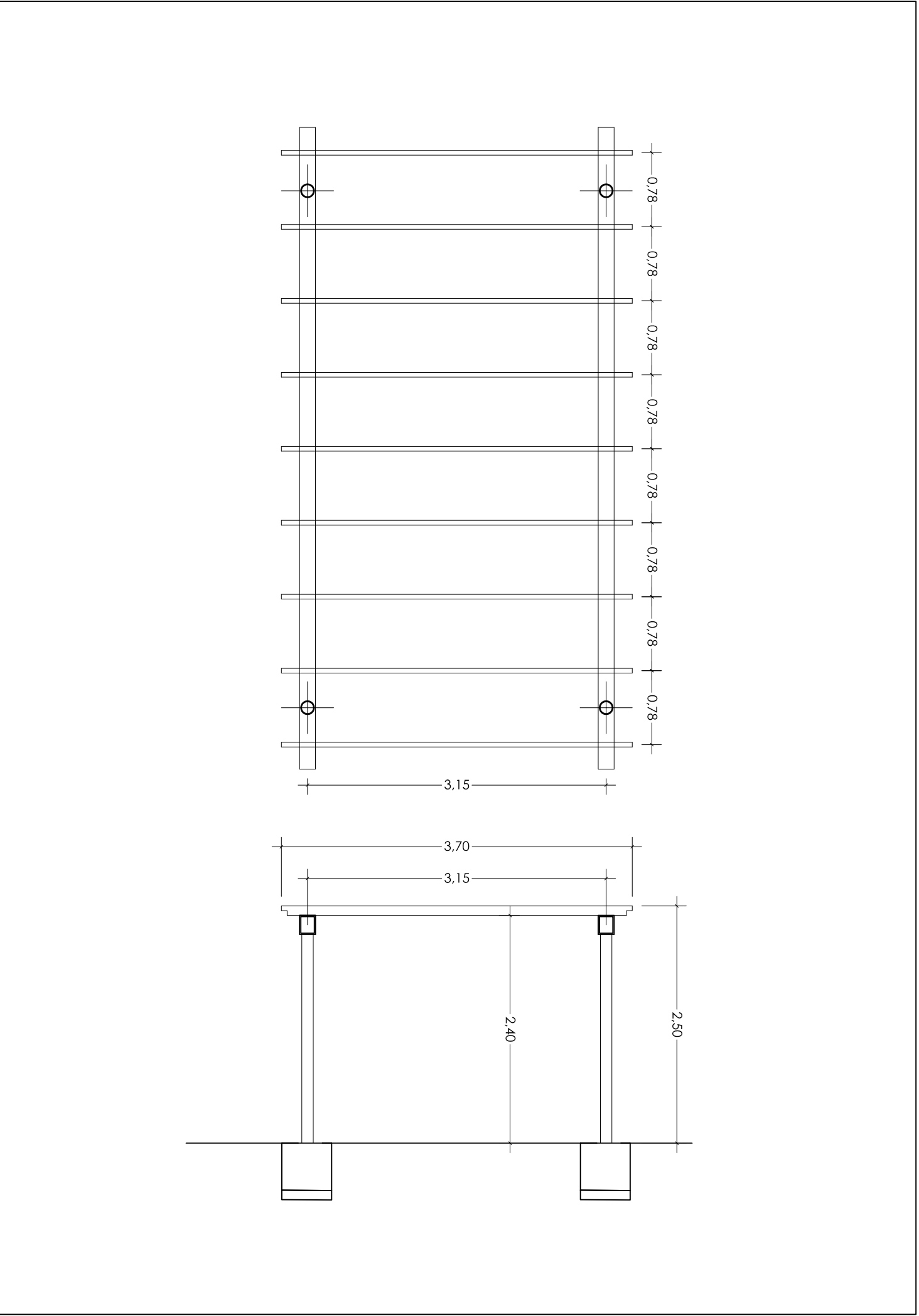
PERGOLA FORMADA POR PERFILERIA DE CHAPA DE ACERO PRELACADA
