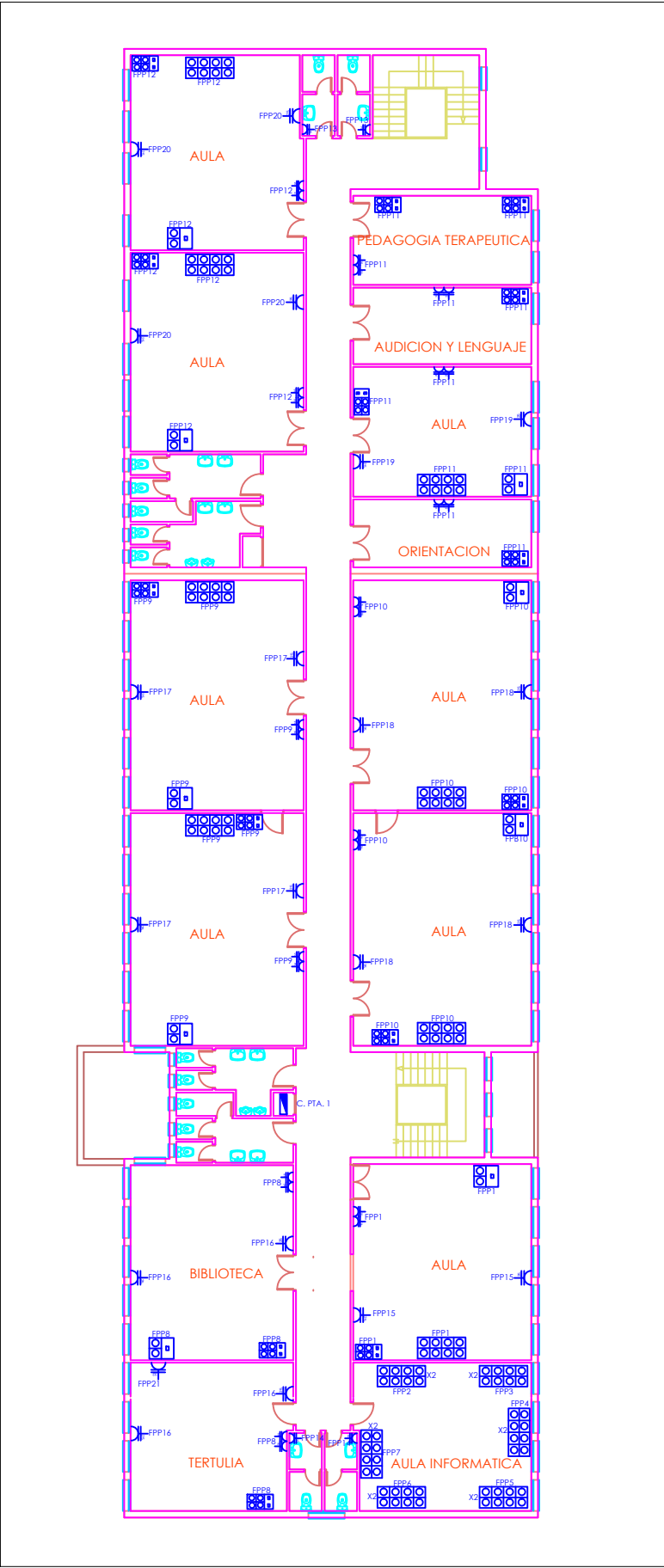
PLANTA PRIMERA
