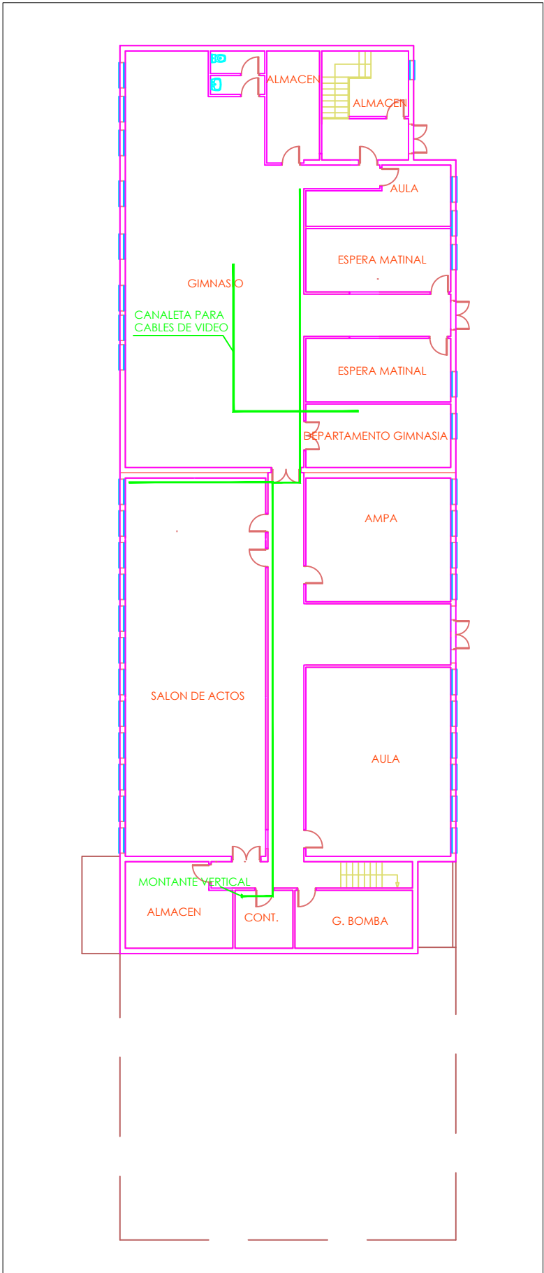
PLANTA SÓTANO
