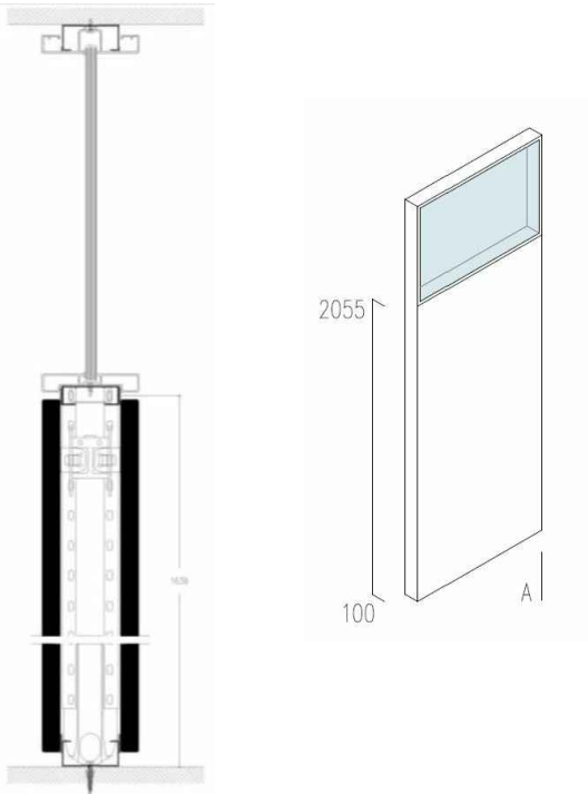
MAMPARA MIXTA CIEGA Y VIDRIO
