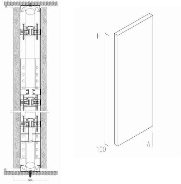
TABIQUE VERTICAL CIEGO
