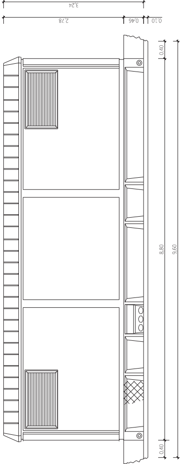
ALZADO POSTERIOR
