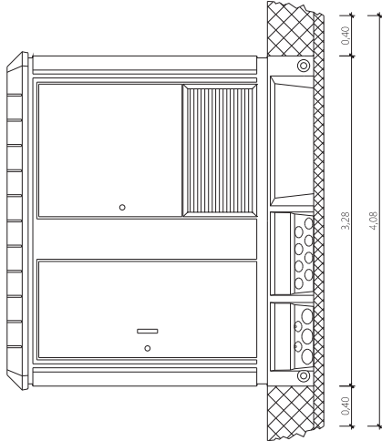
ALZADO FRONTAL
