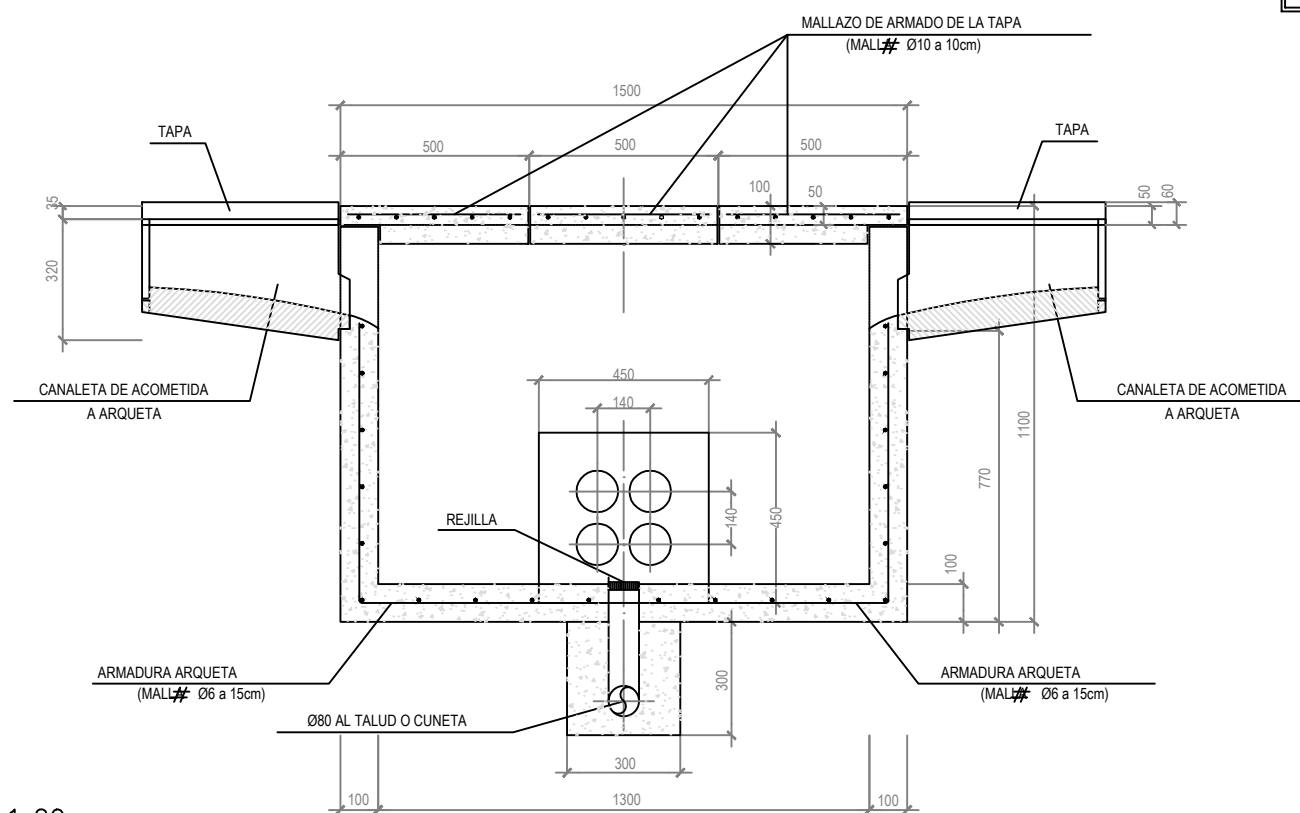
SECCIÓN A-A
