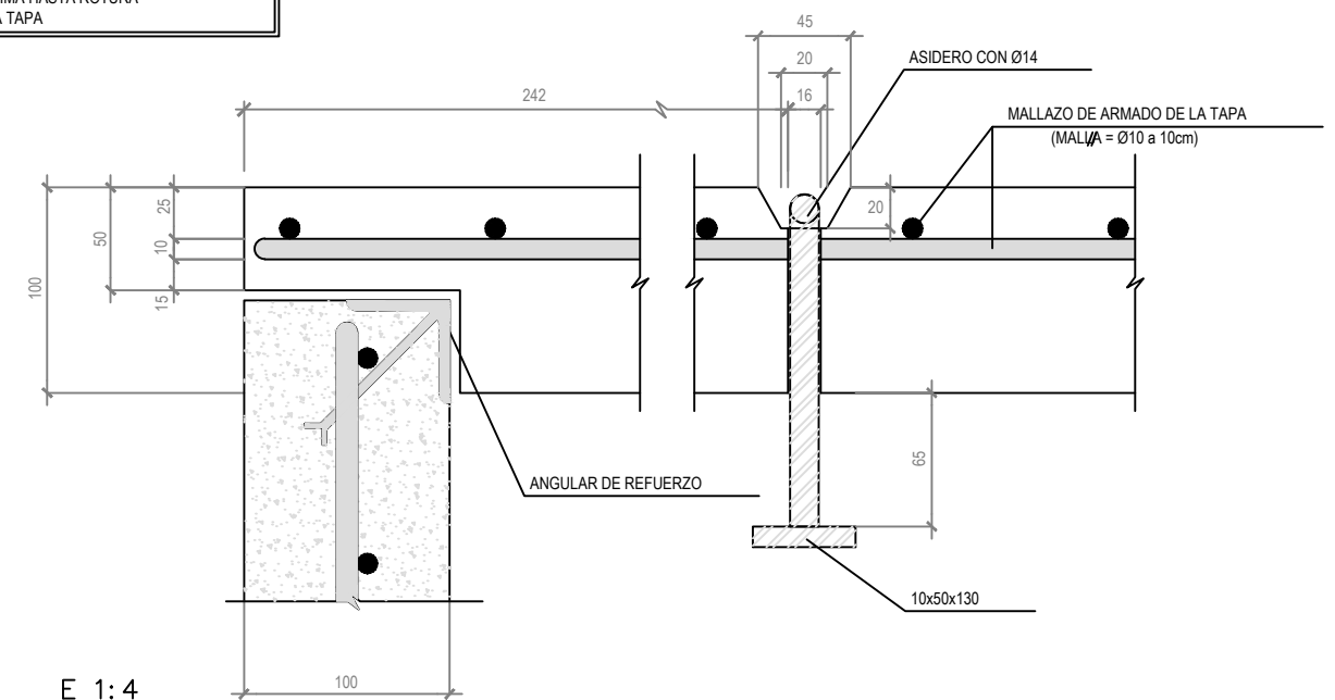
SECCIÓN C-C ( DETALLE DE ASIDERO )
