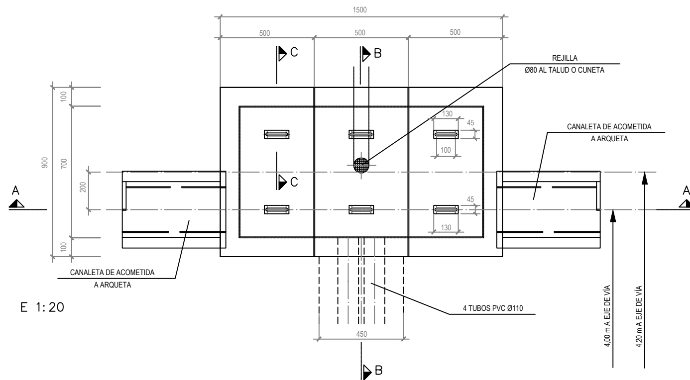
PLANTA
